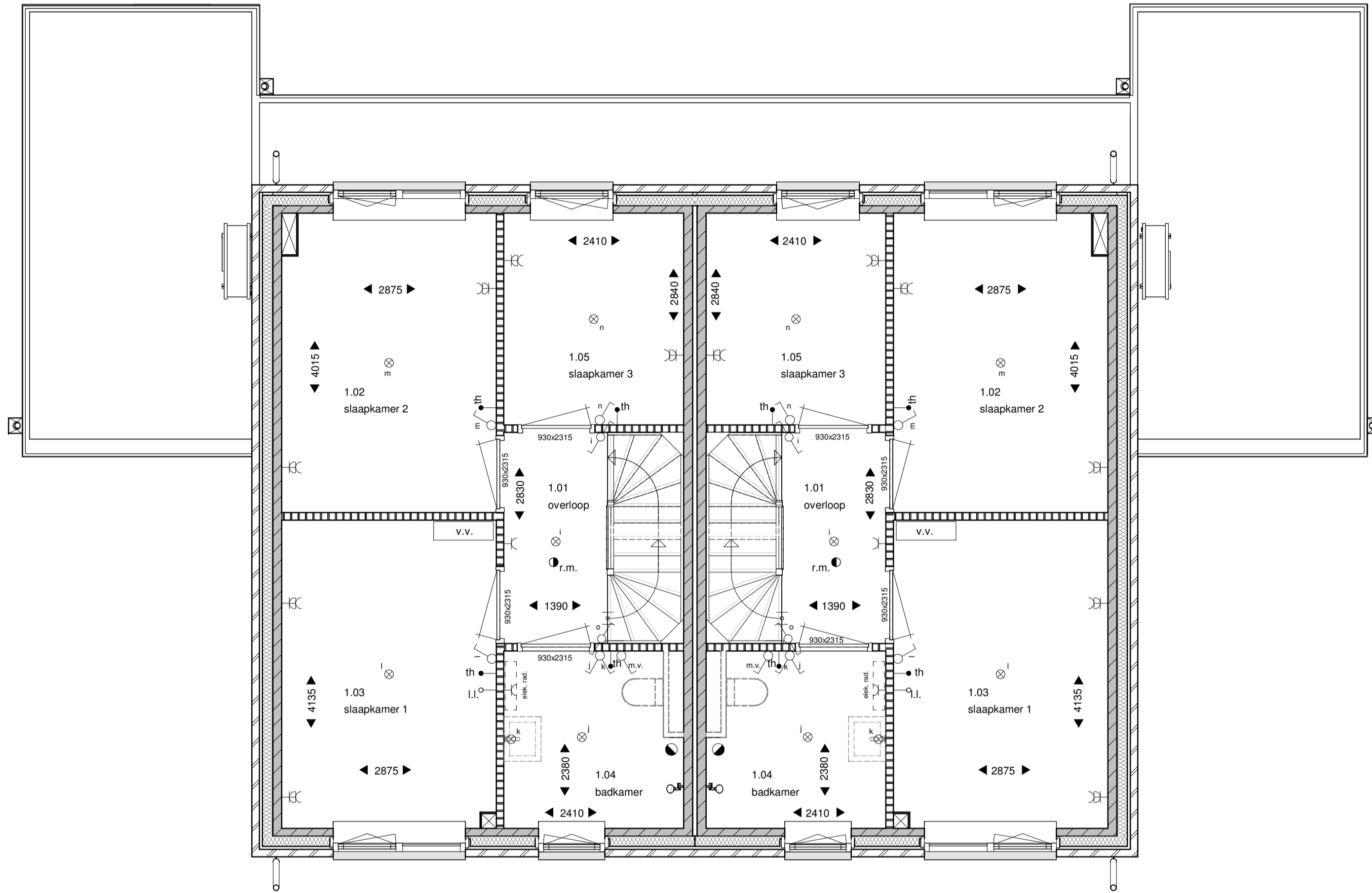
eerste verdieping
