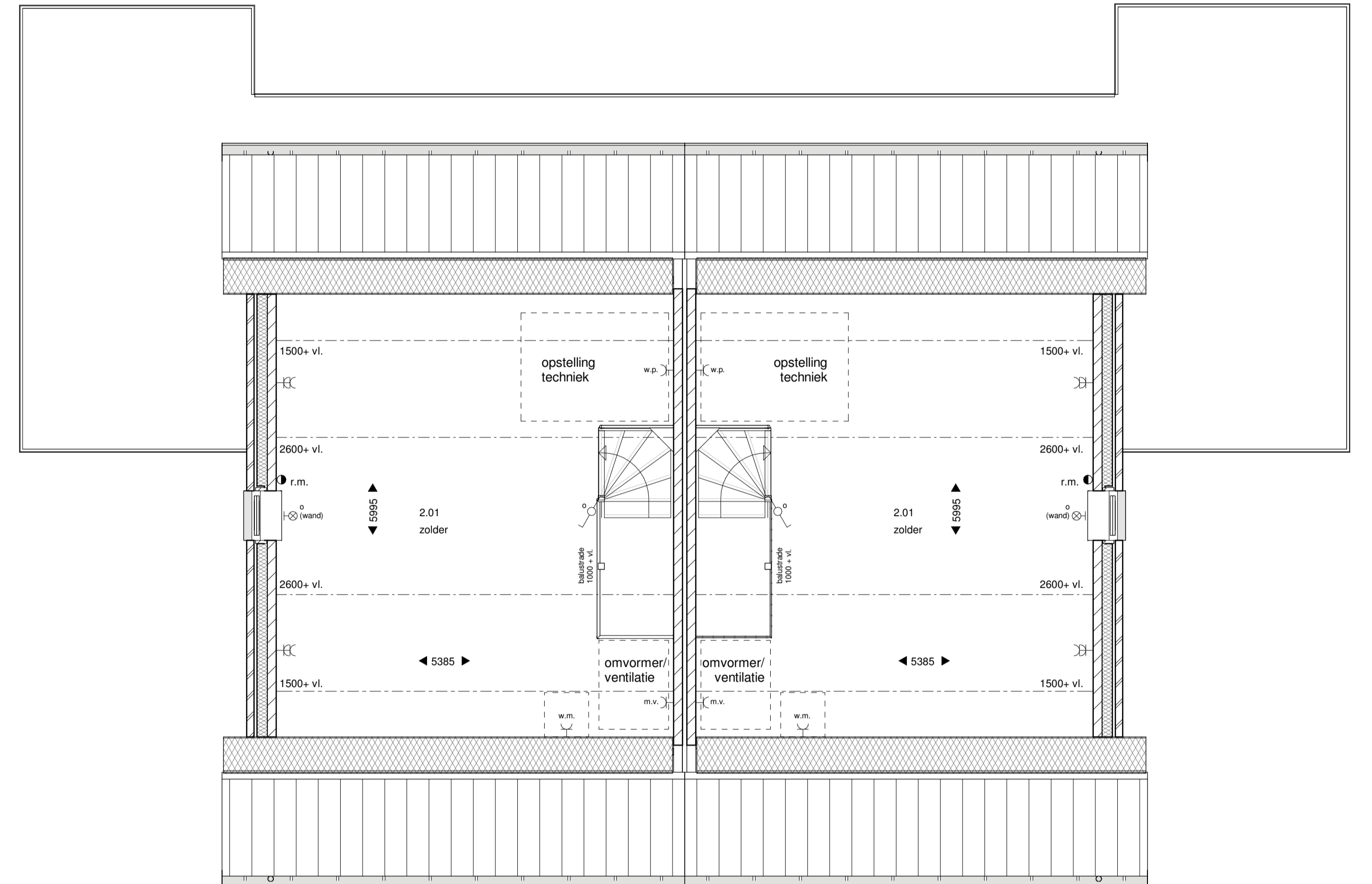
tweede verdieping
